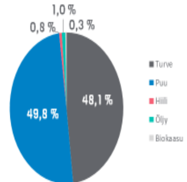
Kaukolämmön tuotannon polttoainejakauma
