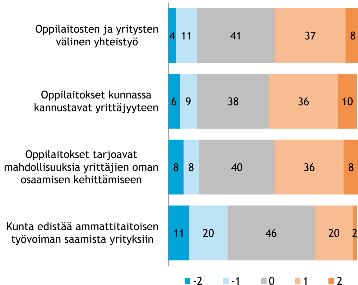
Vastaukset asteikolla, %
